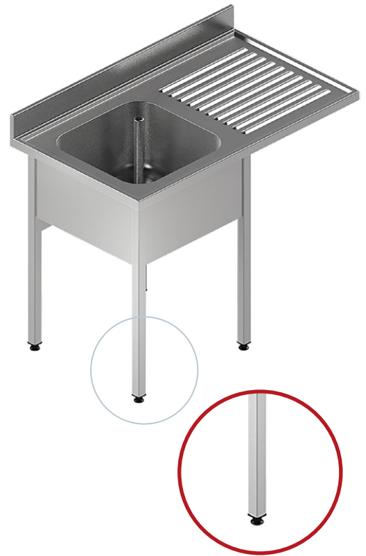
Pieds carrés + vérins de réglages
